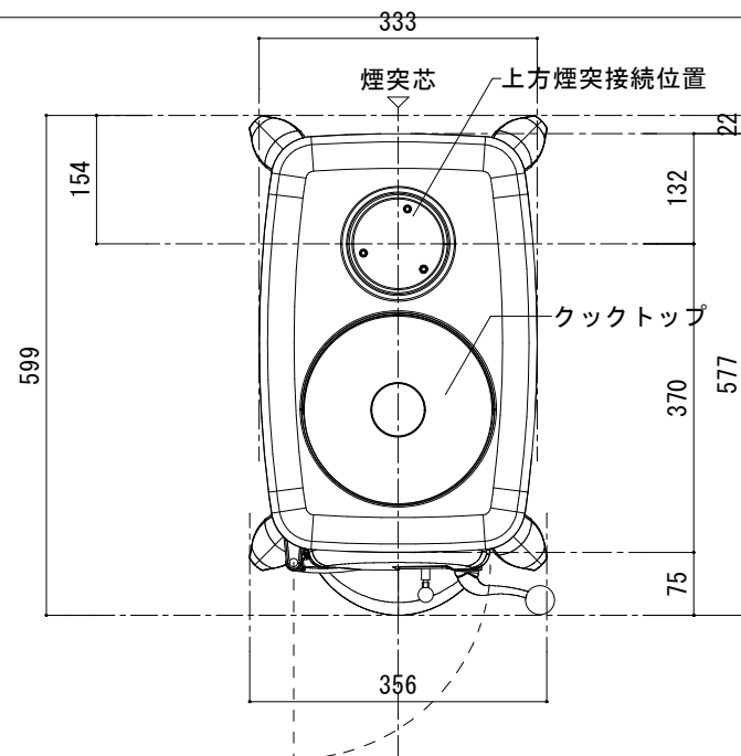
[ 上面図 ]
