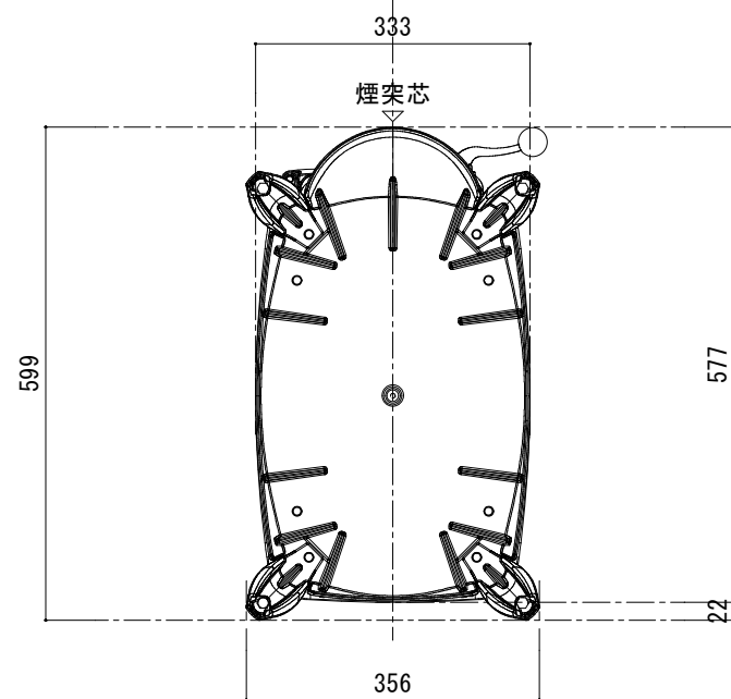
[ 底面図 ]
