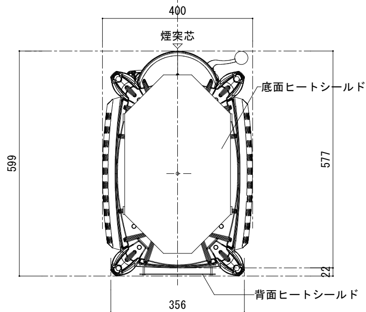
[ 底面図 ]
