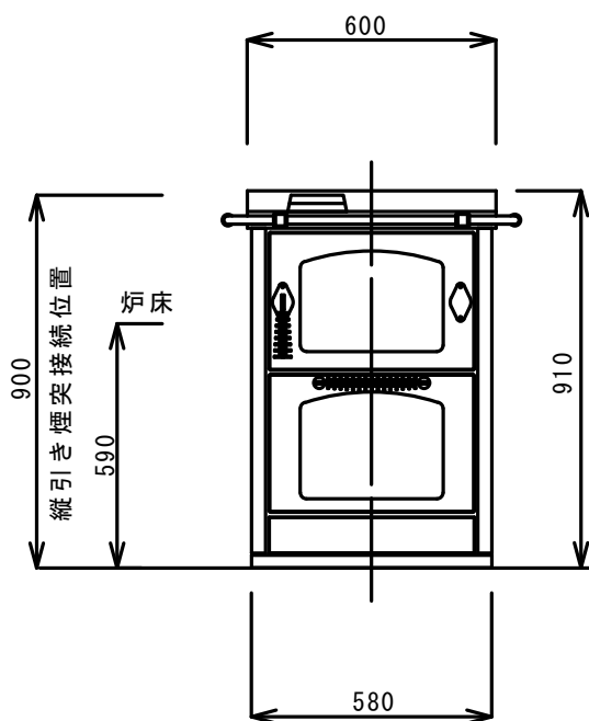
正面図
