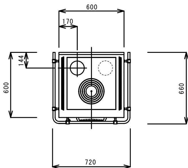
平面図
