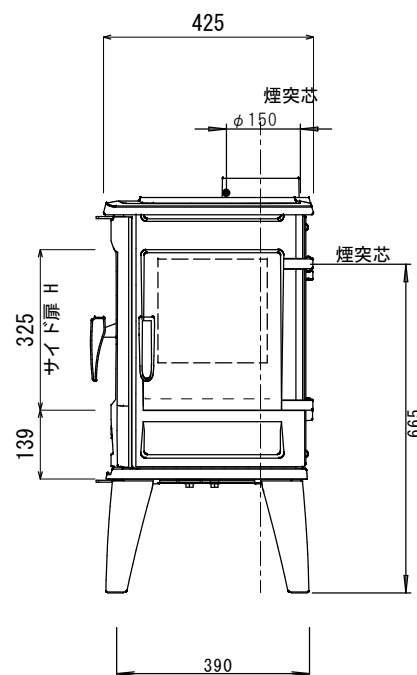
右側面図
