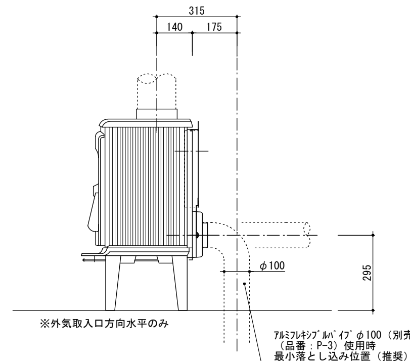
側面図（外気取入口）
