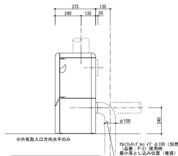
側面図 (外気取入口)
