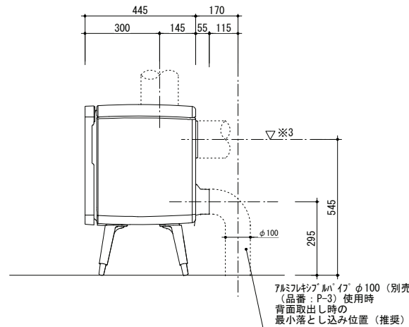
側面図 (外気取入口背面)
