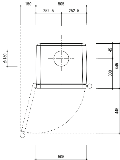
平面図
