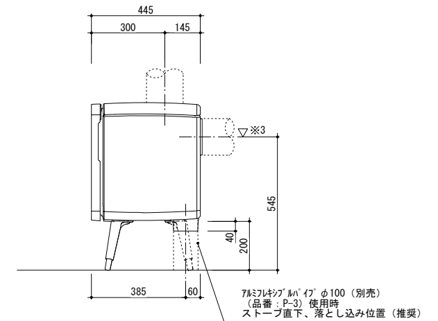
側面図 (外気取入口底面)
