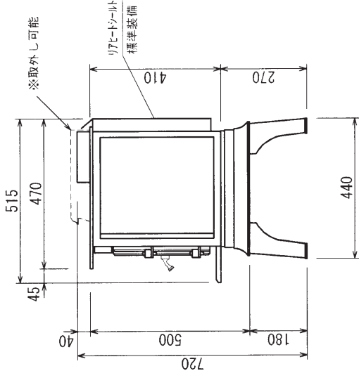
右側面図
