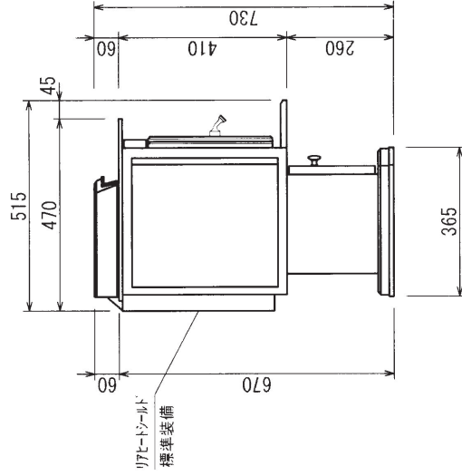
左側面図
