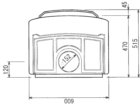
上面図
