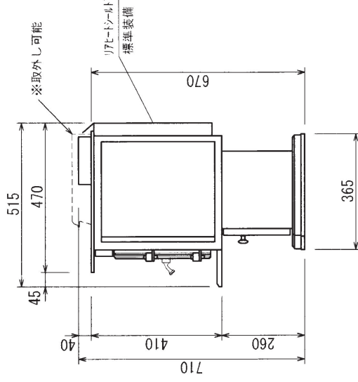
右側面図
