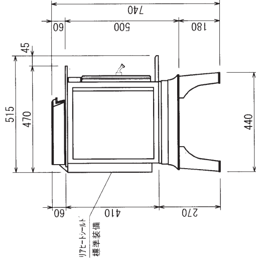
左側面図
