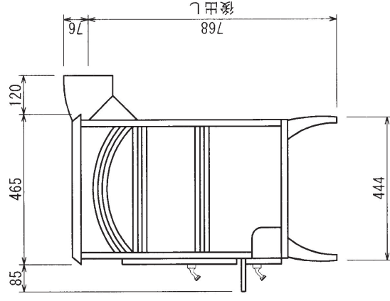
右側面図
