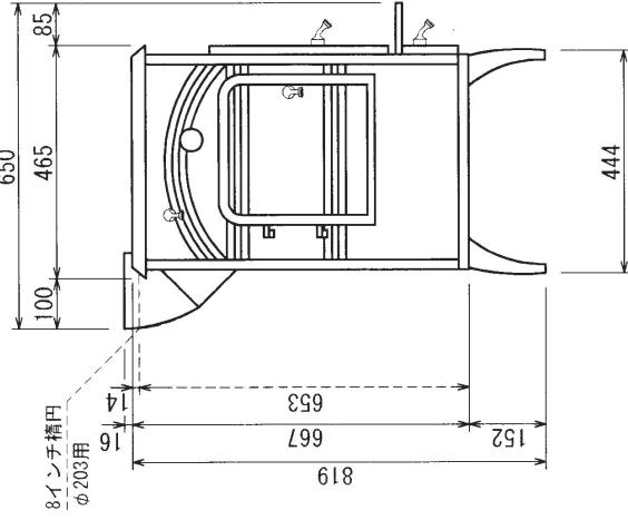
左側面図
