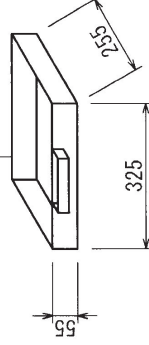
耐熱ガラス
