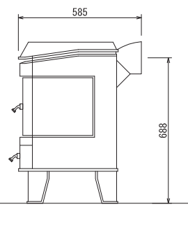
側面図(背面出し)
