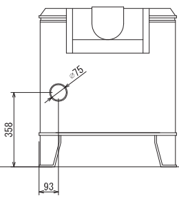
背面図
