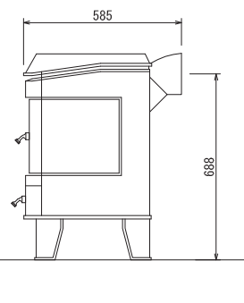
側面図(背面出し)
