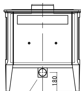
背面図
