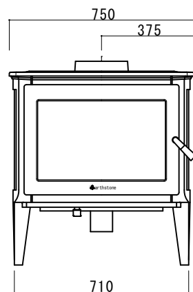
正面図
