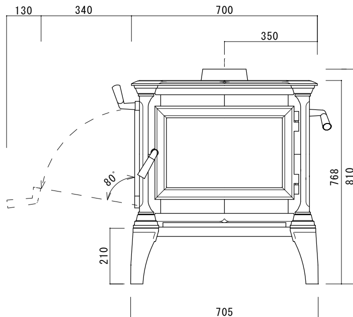
正面図
