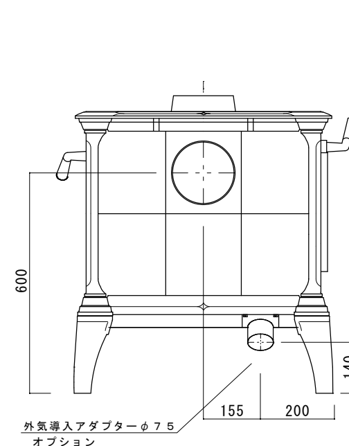
背面図
