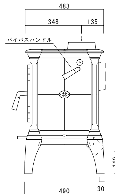
右側面図
