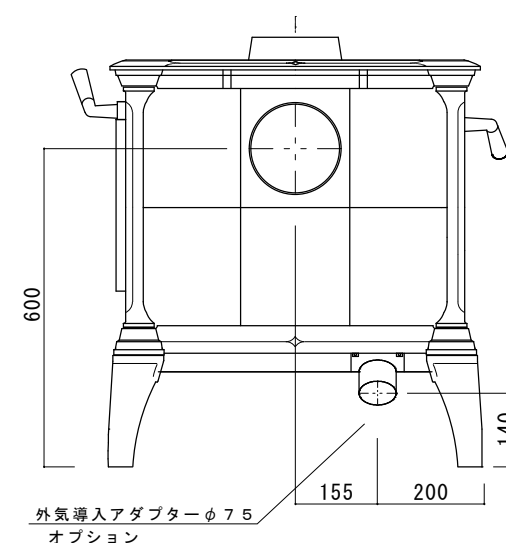
背面図
