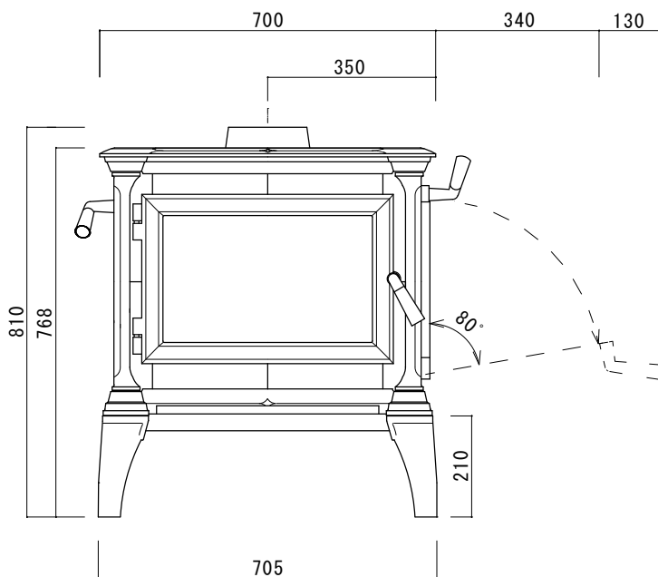
正面図
