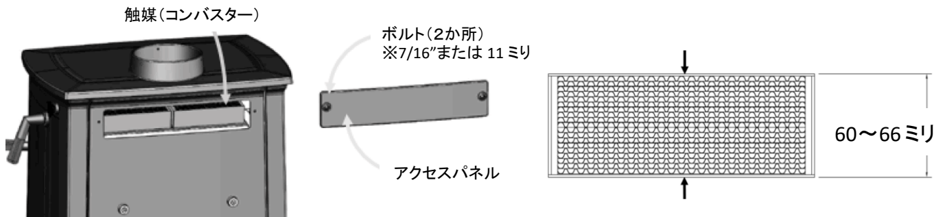
図 8. コンバスター:寸法の目安
