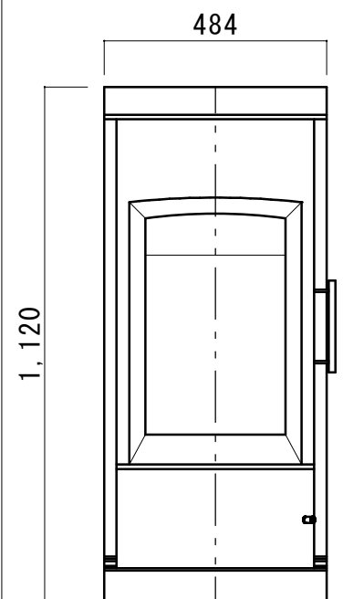
正面図
