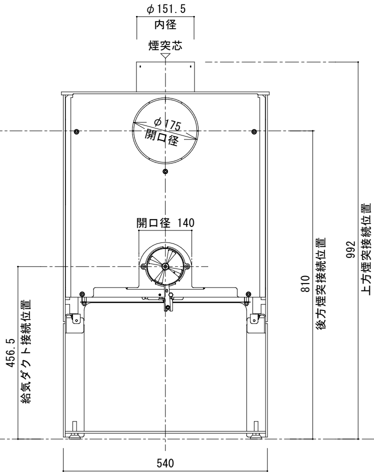
[ 背 面 図 ]
