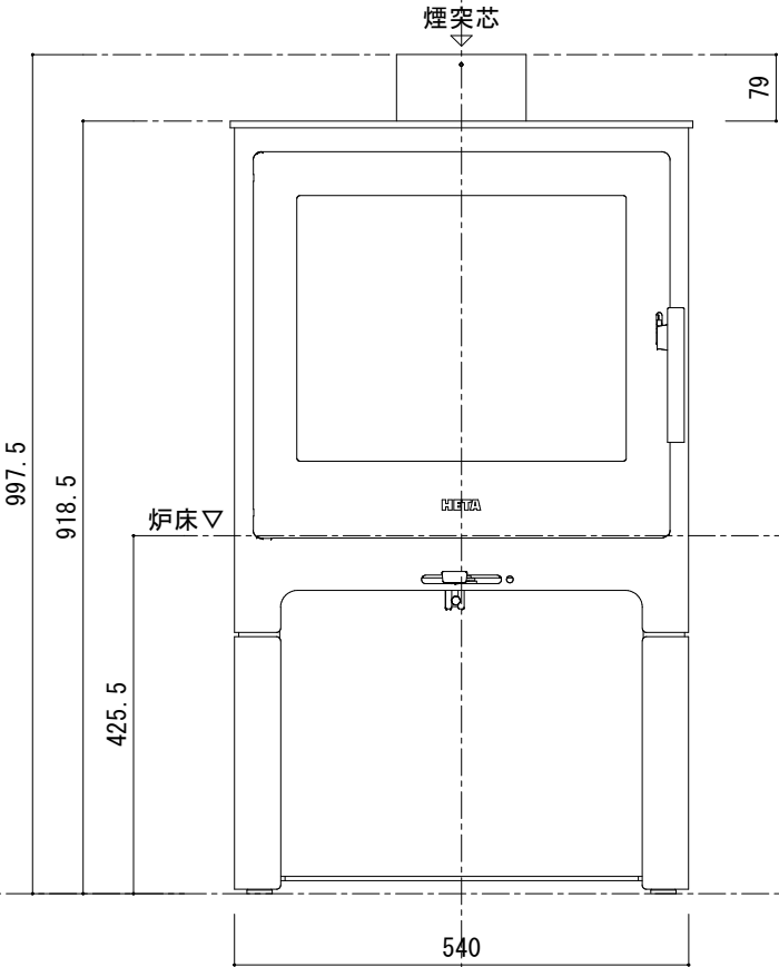
[ 正 面 図 ]
