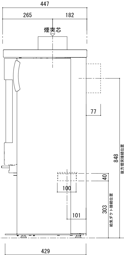
[ 側面図 ]
