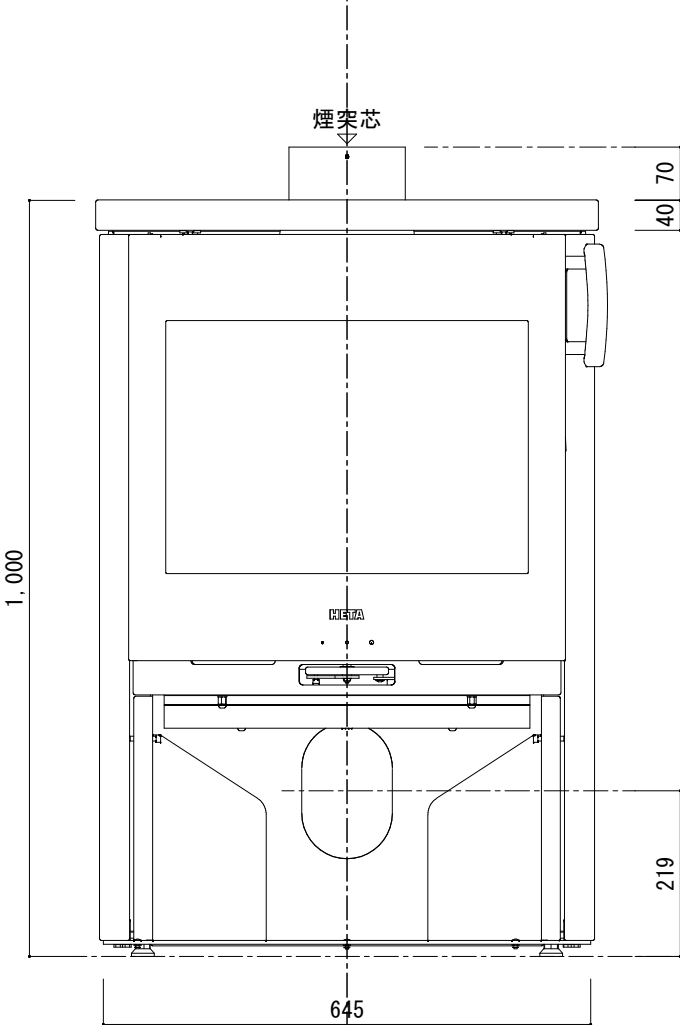
[ 正面図 ]
