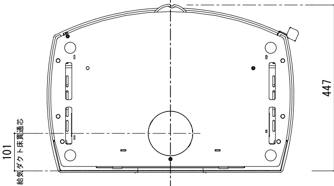
[ 底面図 ]
