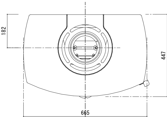
[ 上面図 ]
