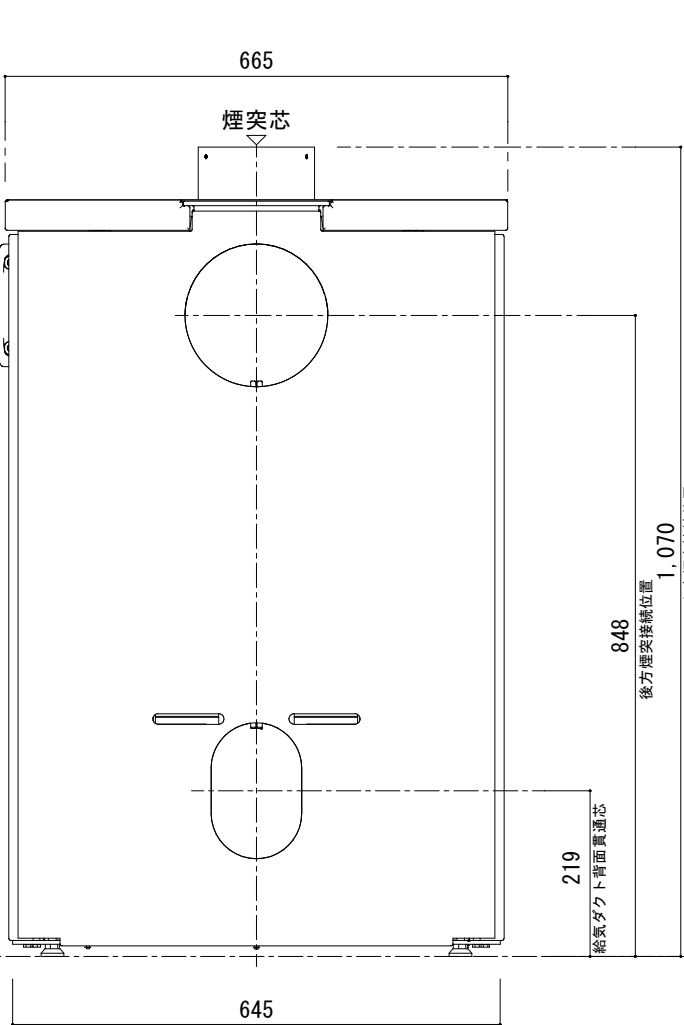
[ 背面図 ]
