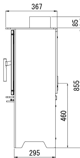
側面図
