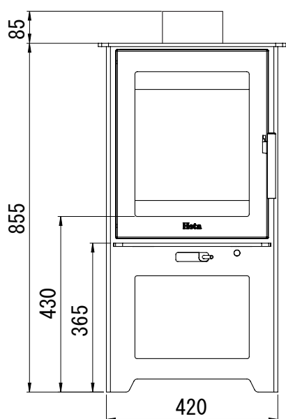
正面図
