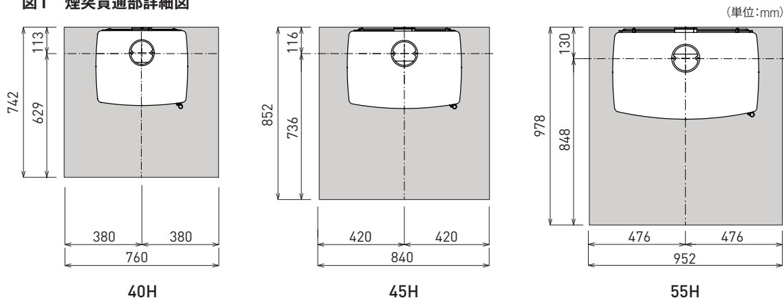
図1 煙突貫通部詳細図
