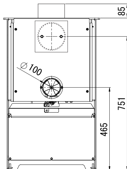
背面図
