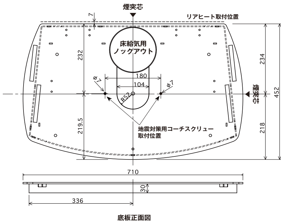
本体ボトムプレート上面図
