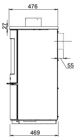
側面図
