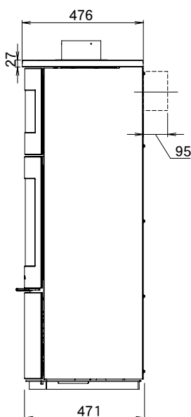
側面図
