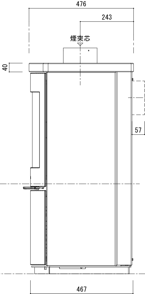
[ 側 面 図 ]
