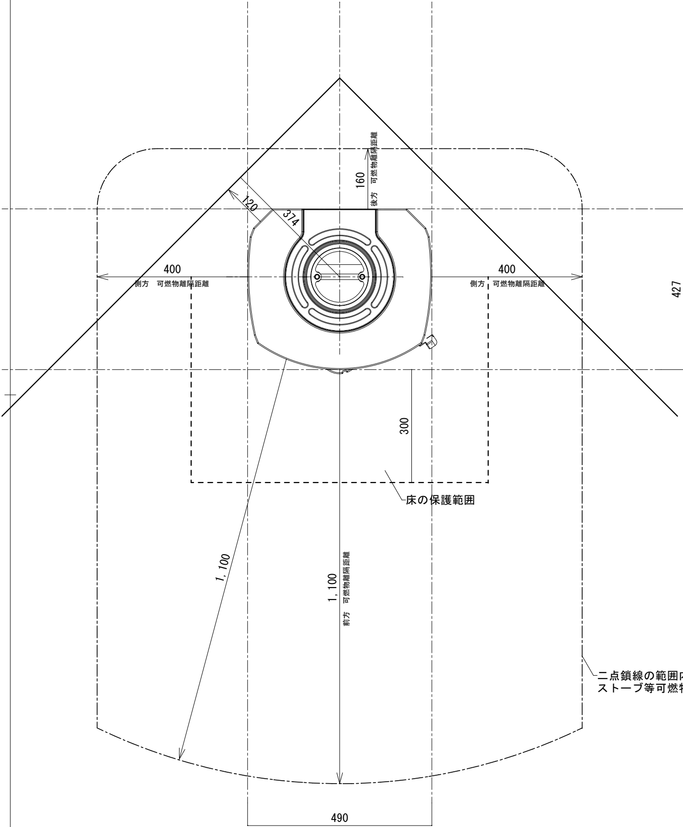
遮熱板なし
