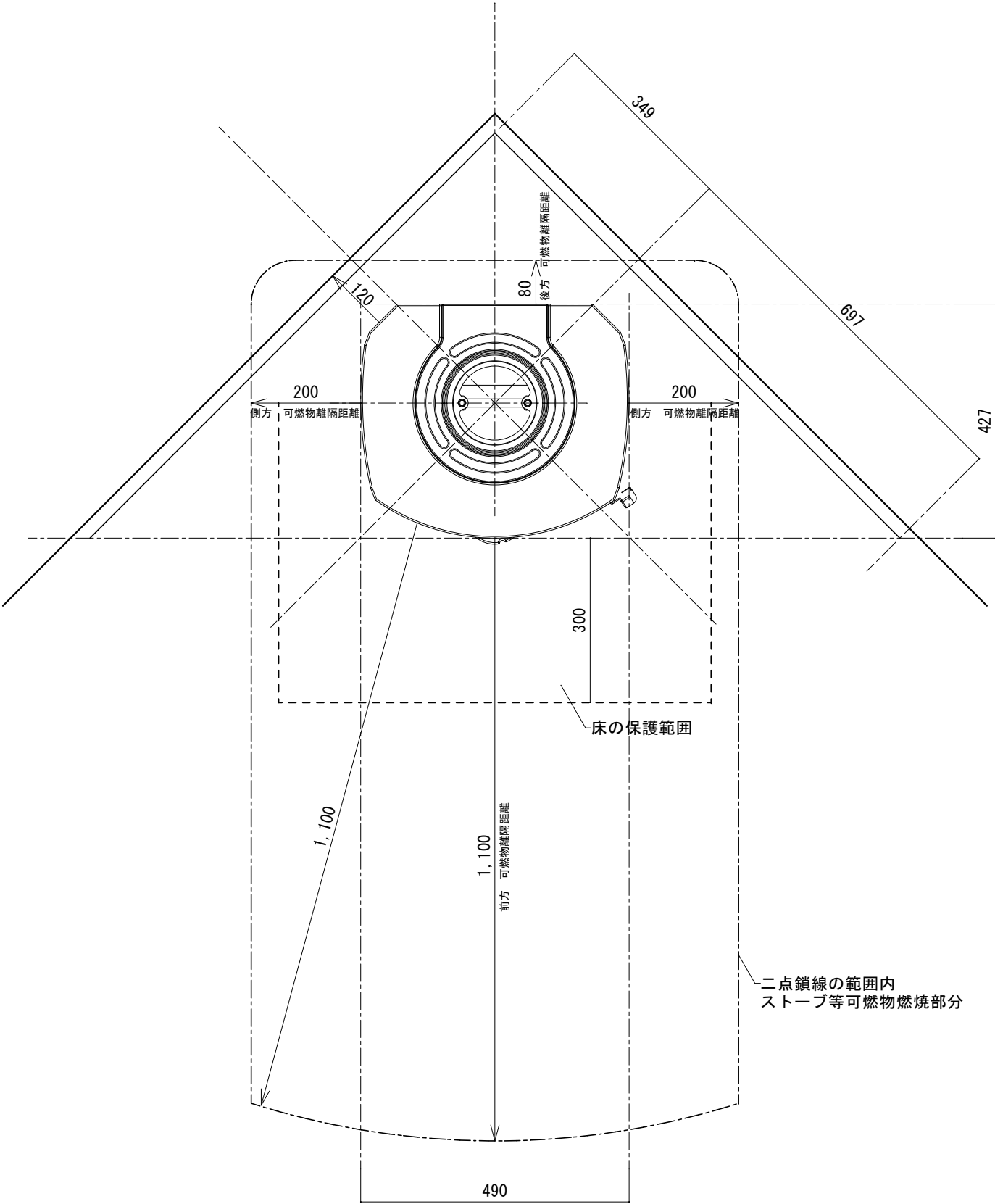
遮熱板あり
