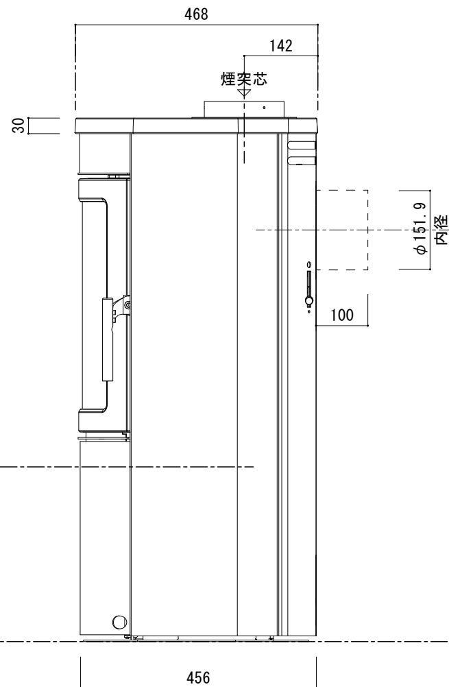
[ 側 面 図 ]
