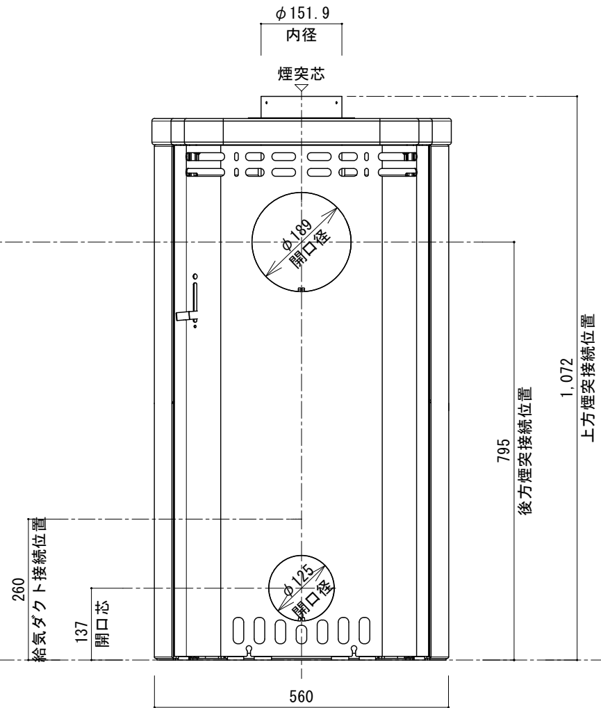
[ 背 面 図 ]
