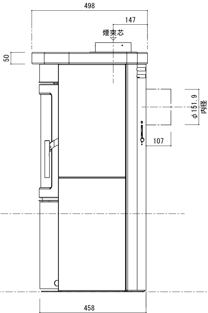
[ 側 面 図 ]
