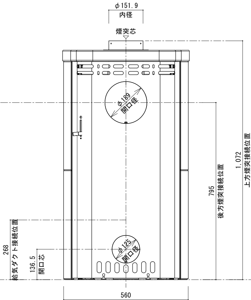
[ 背 面 図 ]
