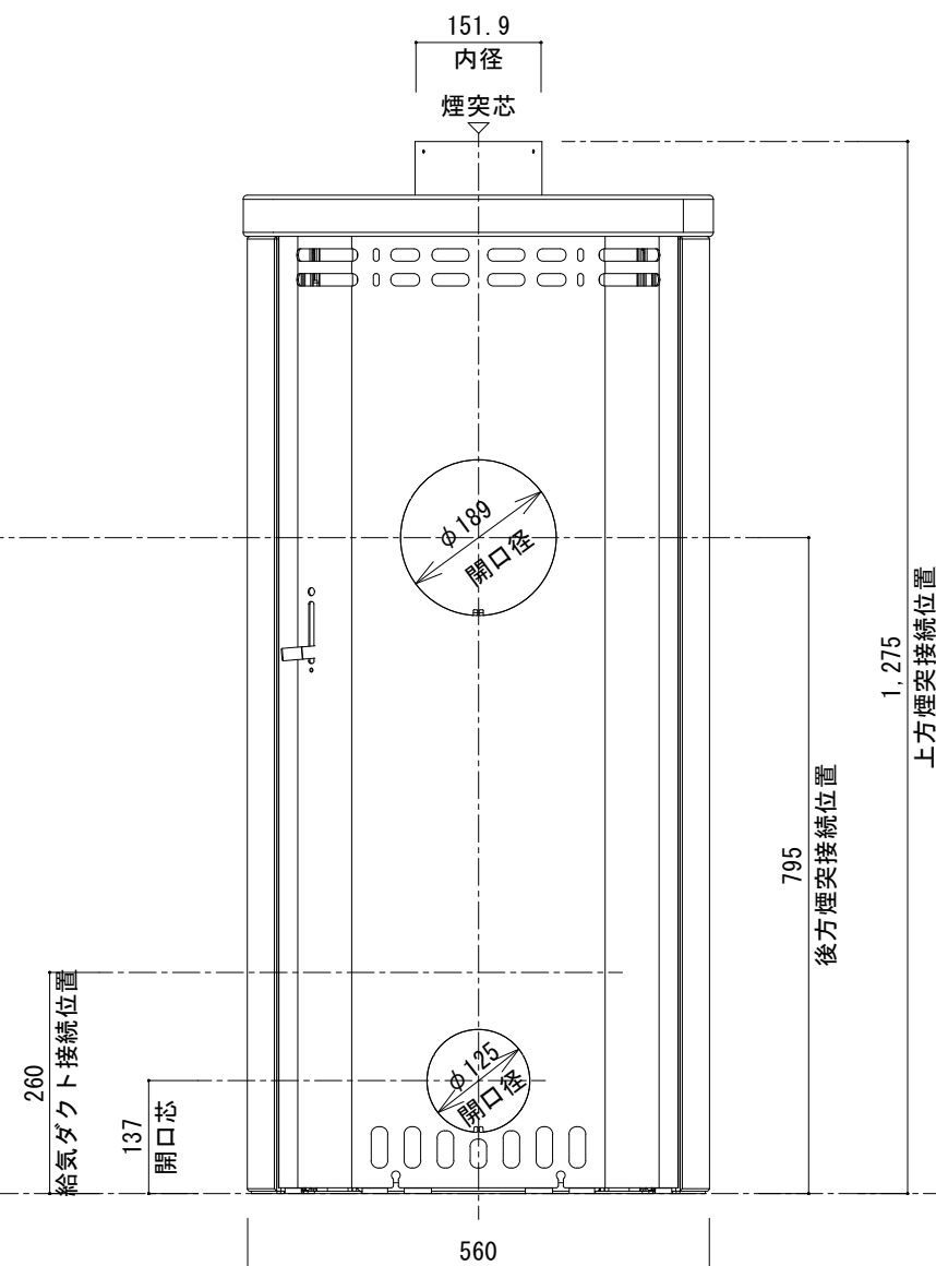
[ 背 面 図 ]
