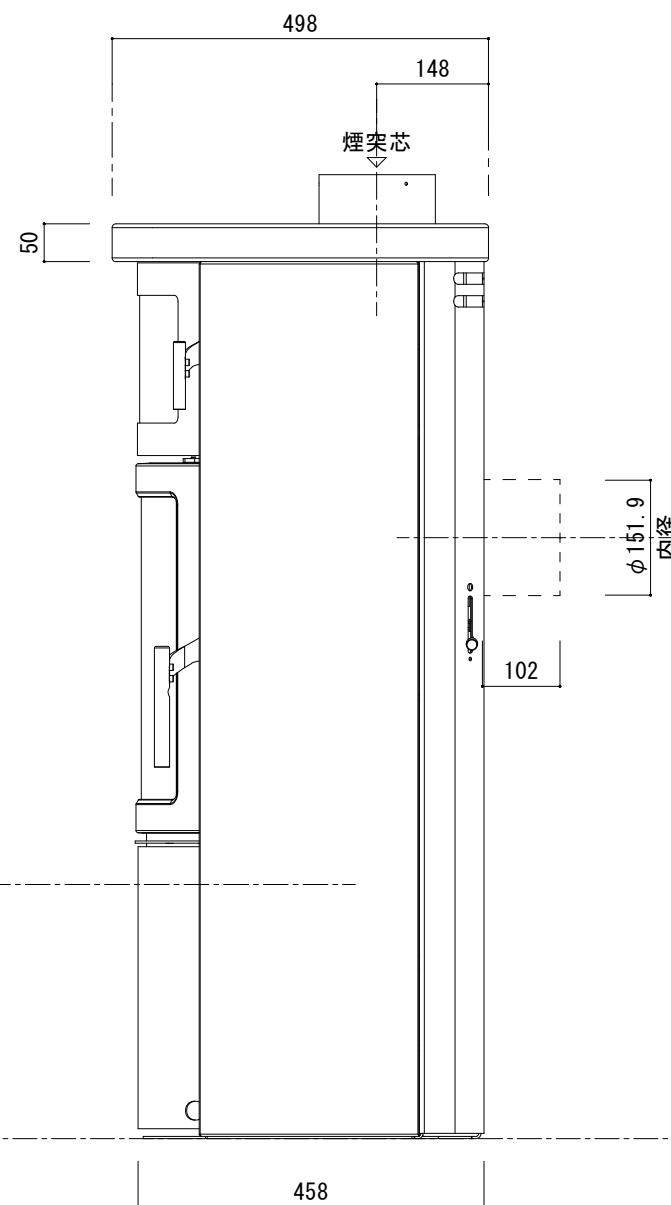
[ 側 面 図 ]
