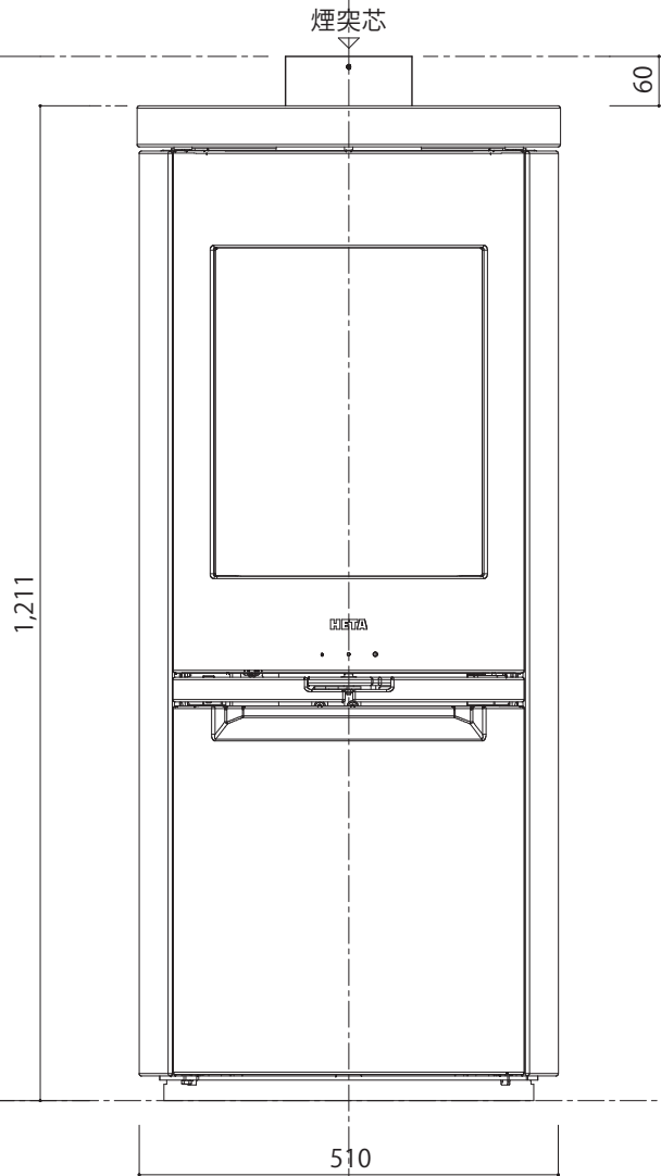
[ 正面図 ]
