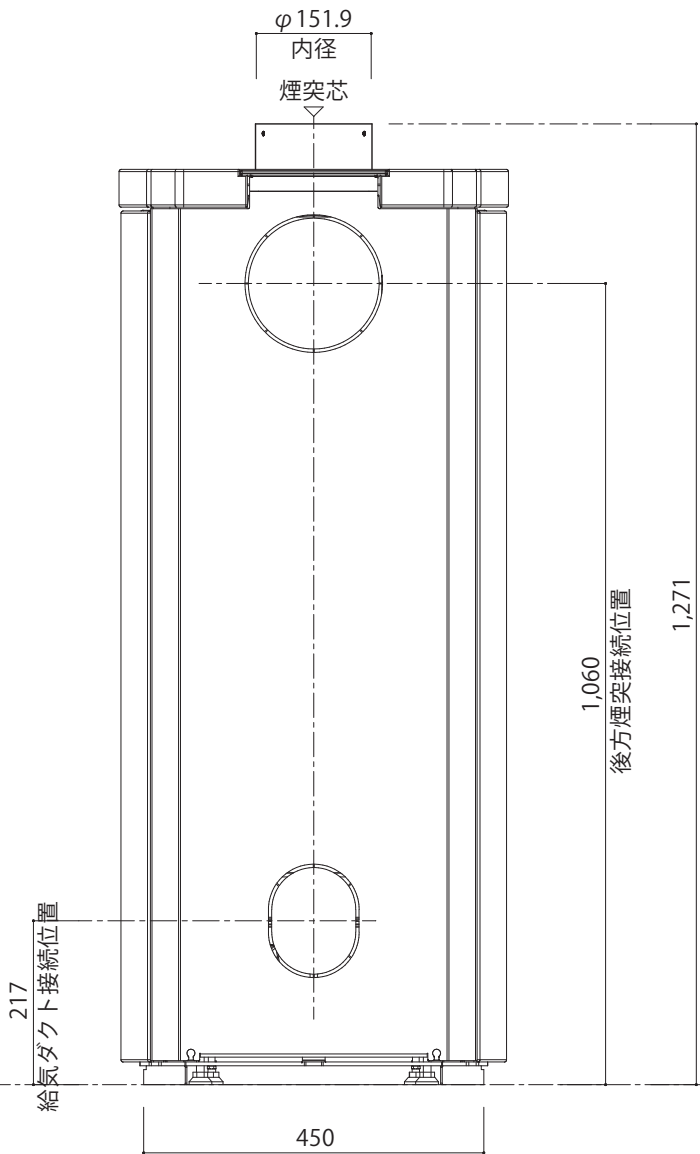
[ 背面図 ]
