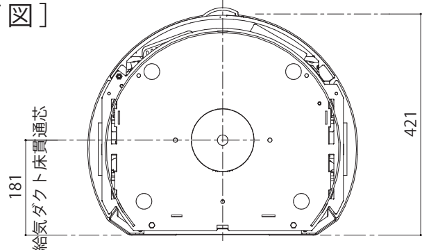
[ 底面図 ]
