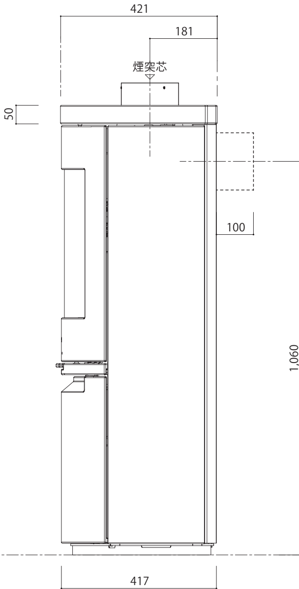
[ 側面図 ]
