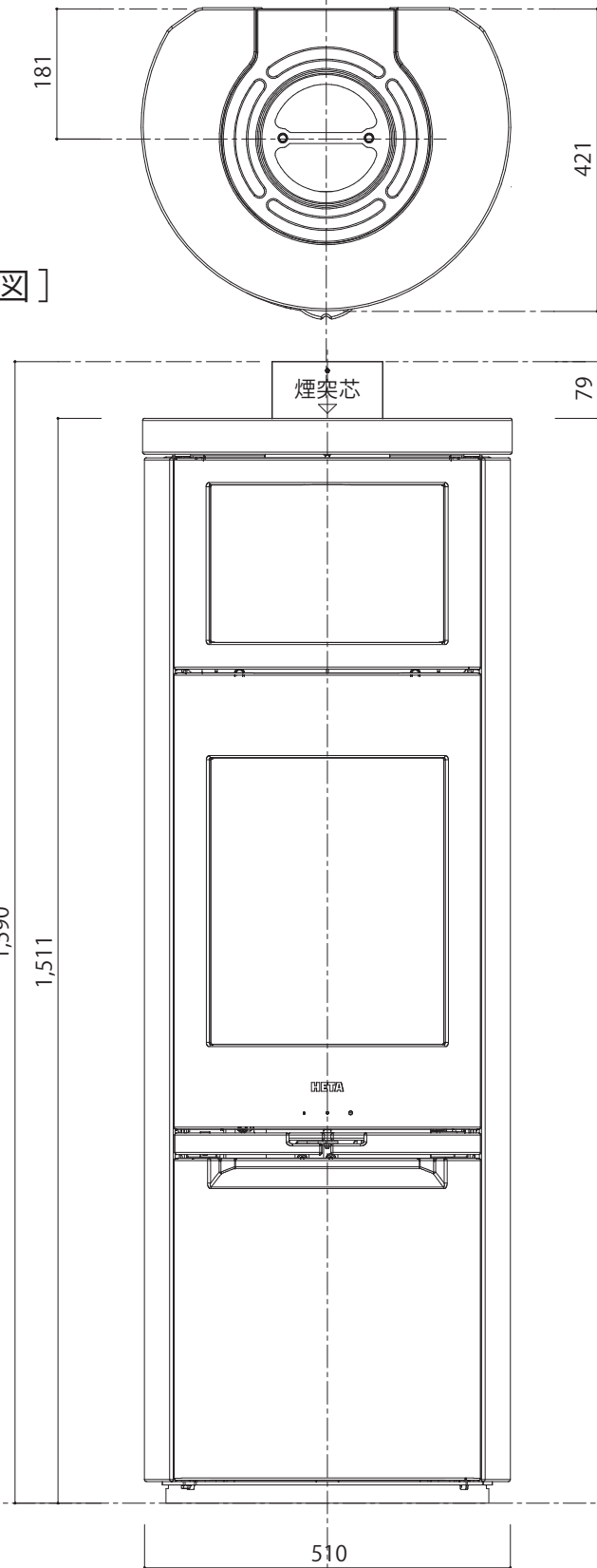
[ 正面図 ]
