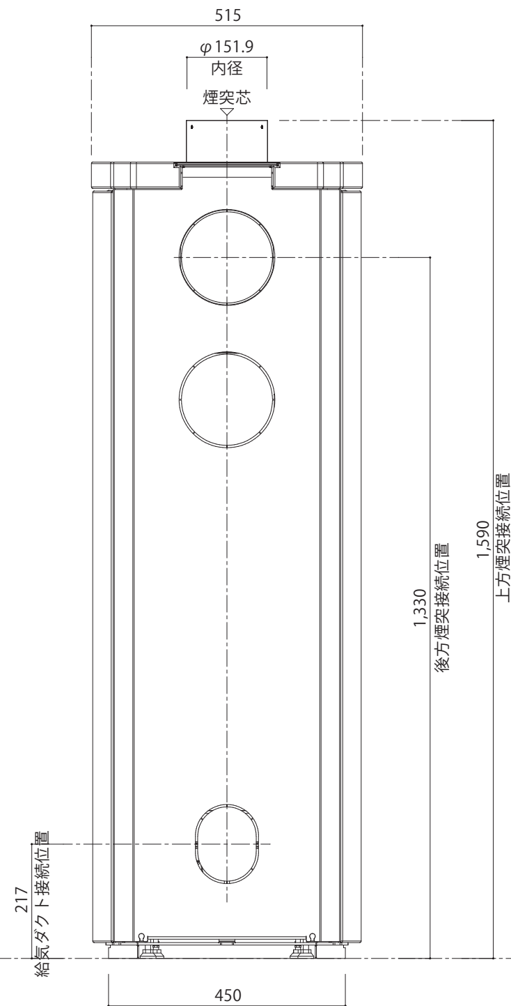
[ 背面図 ]
