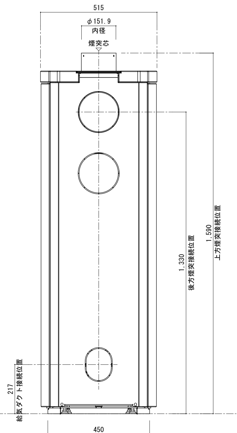
[ 背 面 図 ]
