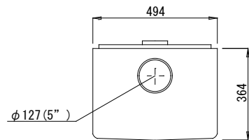
平面図
