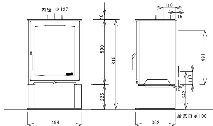
正面図
