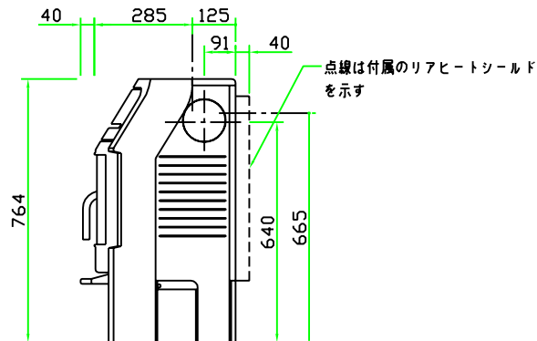
側面図
