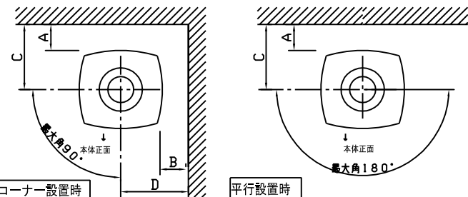
本体離隔距離 F 2 7 3 ターンプレート装備時
