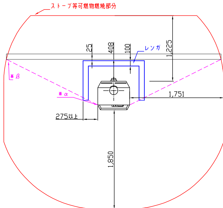
平面図 平行設置 レンガ積み
