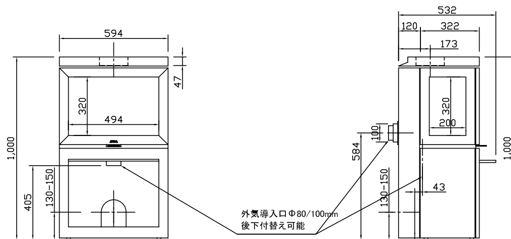
正面図
