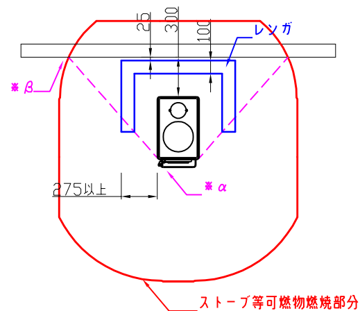
平面図 平行設置 レンガ積み
