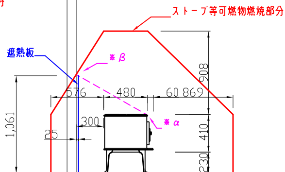
側面図 平行設置
