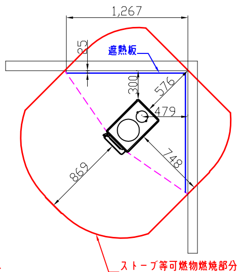
平面図 コーナー設置
