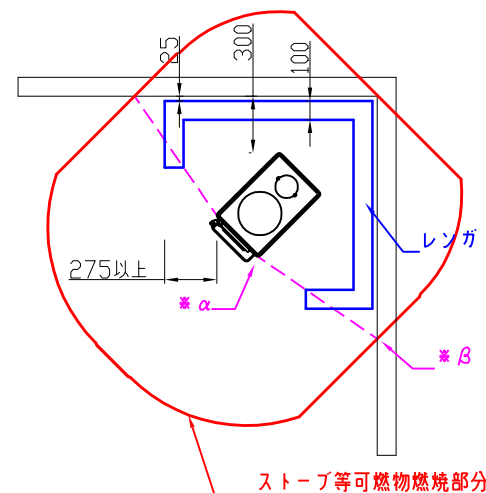
平面図 コーナー設置 レンガ積み
