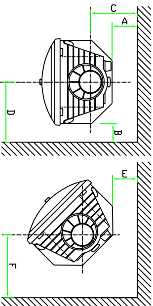
本体離隔距離図
