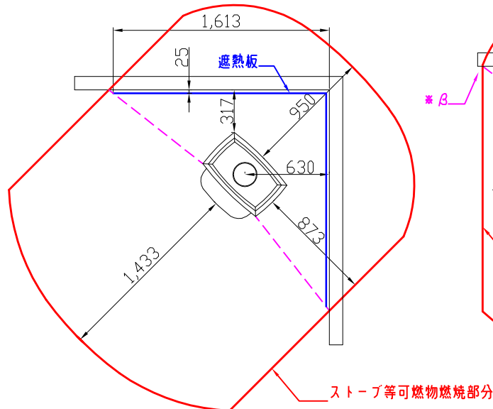
平面図 コーナー設置
