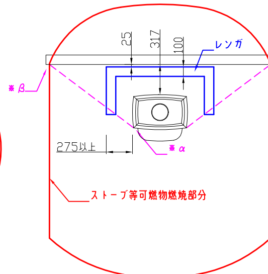
平面図 平行設置 レンガ積み
