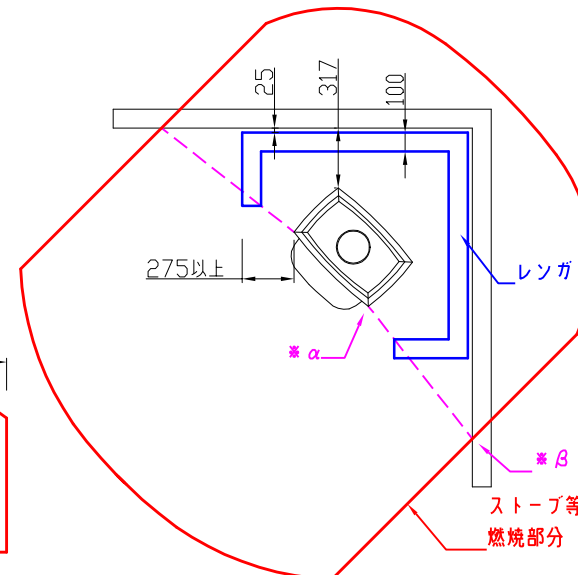
平面図 コーナー設置 レンガ積み
