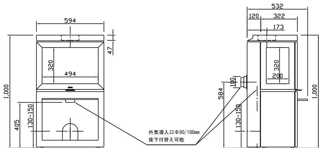
正面図
