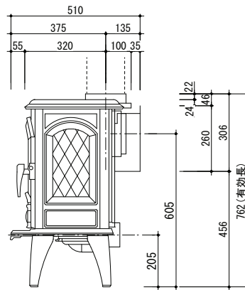
側面図
