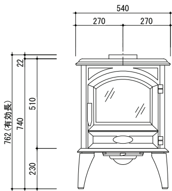
正面図
