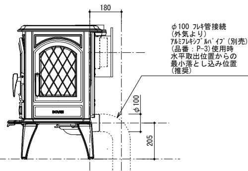
側面図 (外気取入口)
