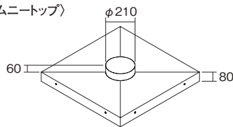
〈取付架台〉
