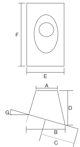
〈30°ユニバーサルフラッシング〉
