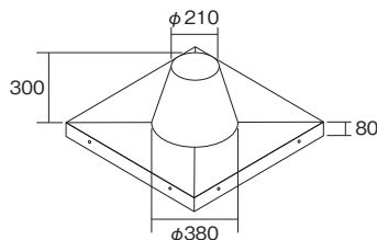
〈チムニートップカラー付〉
