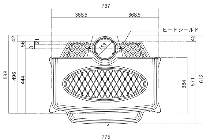
上面図
