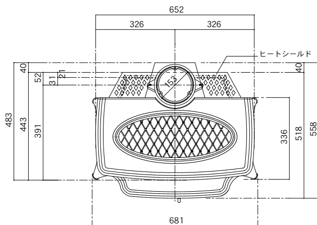
上面図
