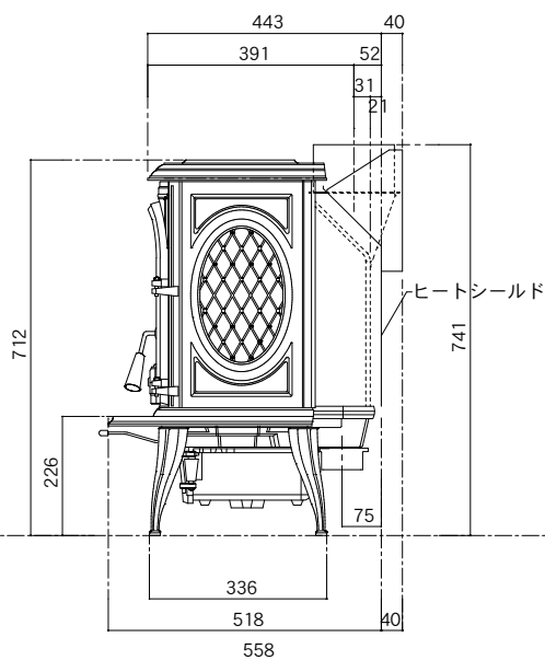
側面図
