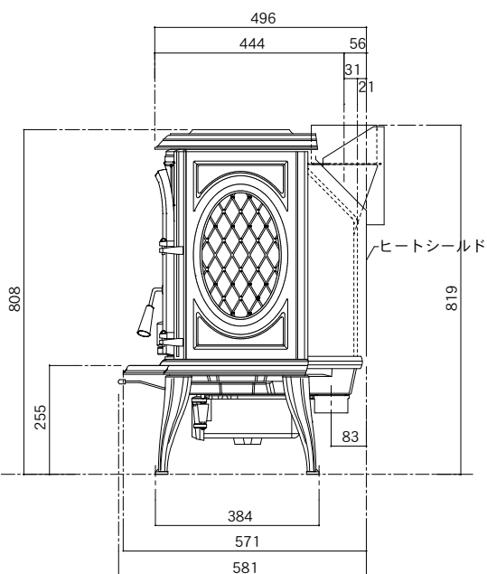
側面図
