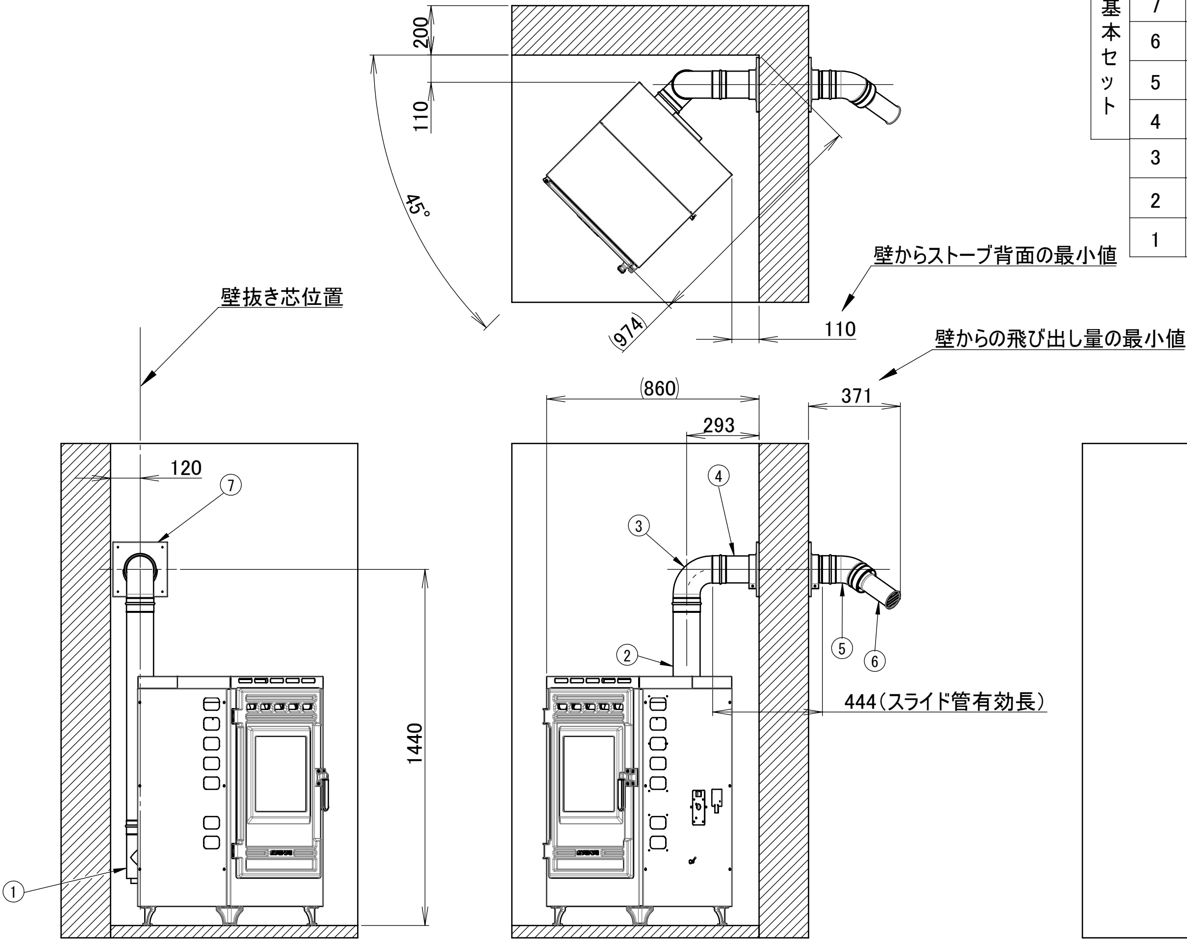
SS-10 室内立上(コーナー右) 給排気管施工図
