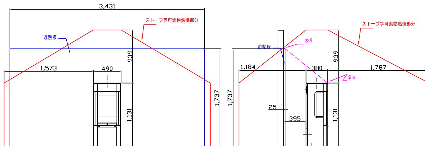
側面図 平行設置
