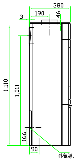
側面図
