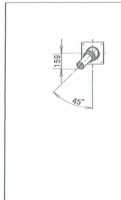
SS-10 室内立上(コーナー右) 給排気管施工図
