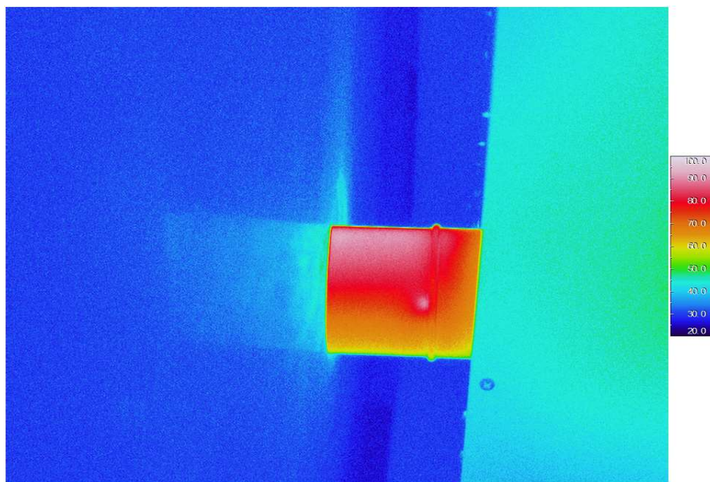
背面の測定時の熱画像
