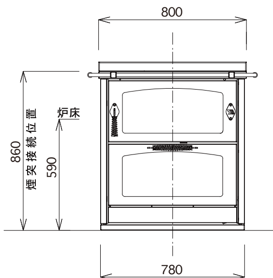
正面図
