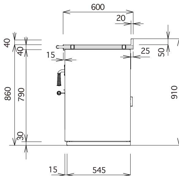
側面図
