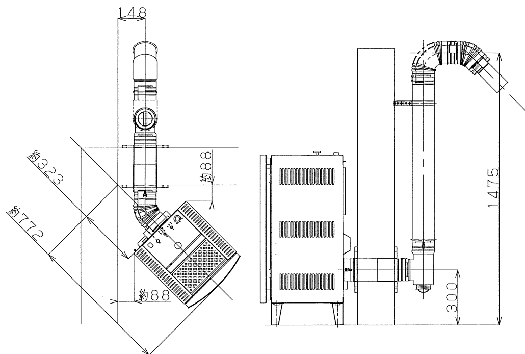
PE-6設置図
